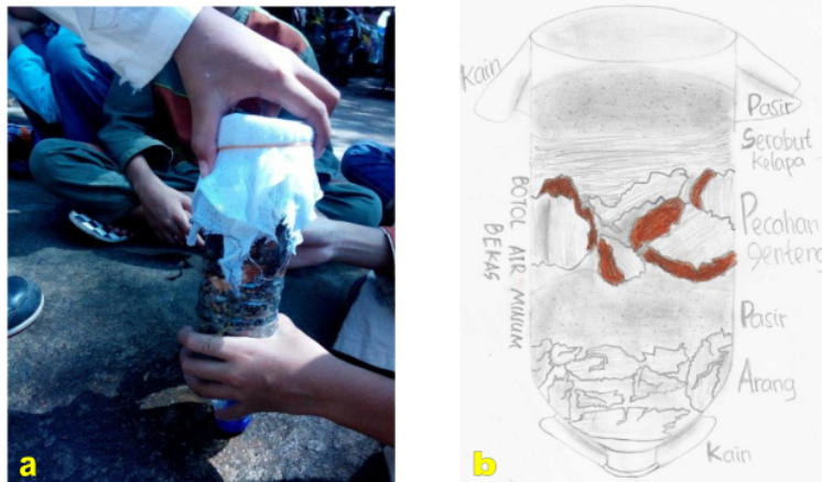
Gambar 1. Media Penjernihan Air Secara Sederhana (a) Hasil dari Peserta (b) Gambaran Alat Penjernihan Sederhana
