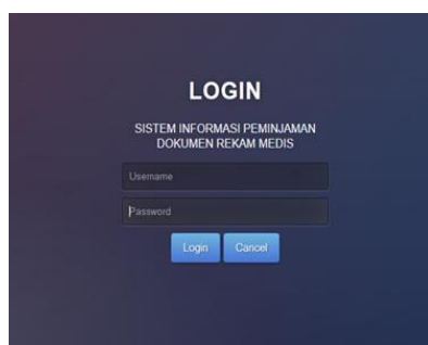
Gambar 2. Menu login
