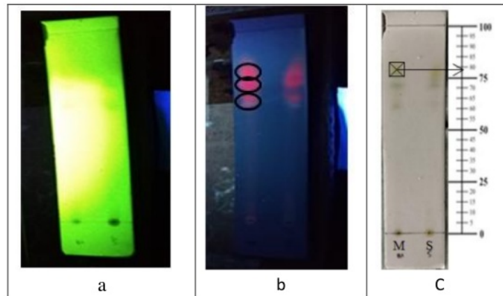
Gambar 1. Profil KLT Herba Daun Gatal. Eluen yang digunakan adalah toluene : etil asetat : asam formiat (5:4:1). a. profil KLT di bawah sinar UV 254 nm. b. profil KLT di bawah sinar UV 366 nm. c. profil KLT setelah diberi penampak bercak uap ammonia.
